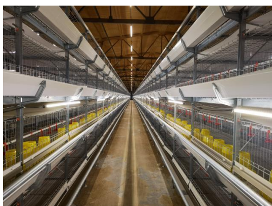
四层笼养设备
