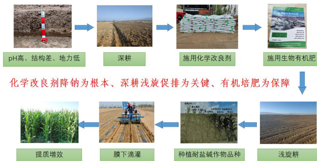
内陆盐碱地降钠促排提质增效技术流程图
